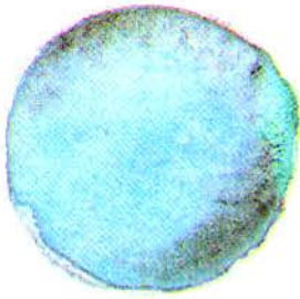
Нептун
