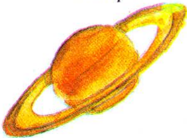
Сатурн
